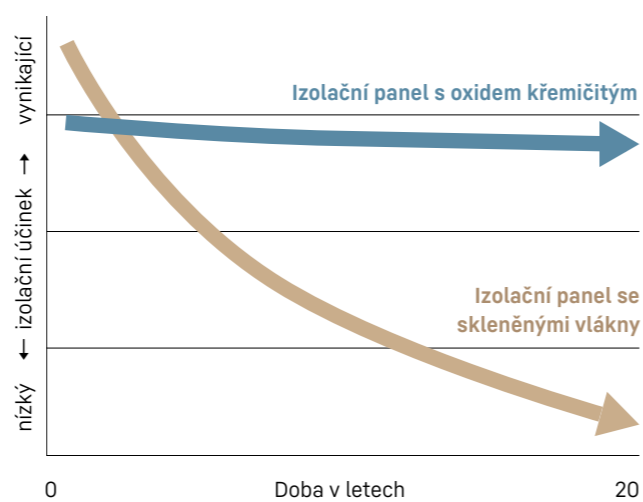
Izolační účinek vakuových panelů
